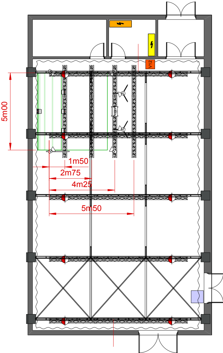
Topview
