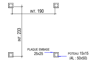
DÉTAIL D'IMPLANTATION DES POTEUX SOUS-SOL ECH : 1CM = 1M
