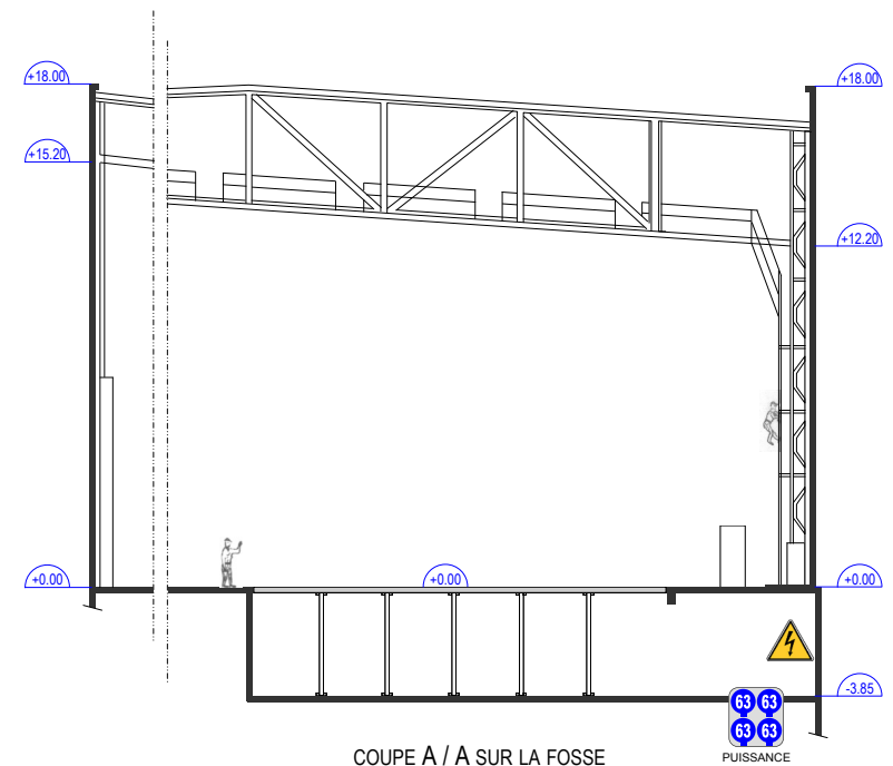
COUPE A / A SUR LA FOSSE
