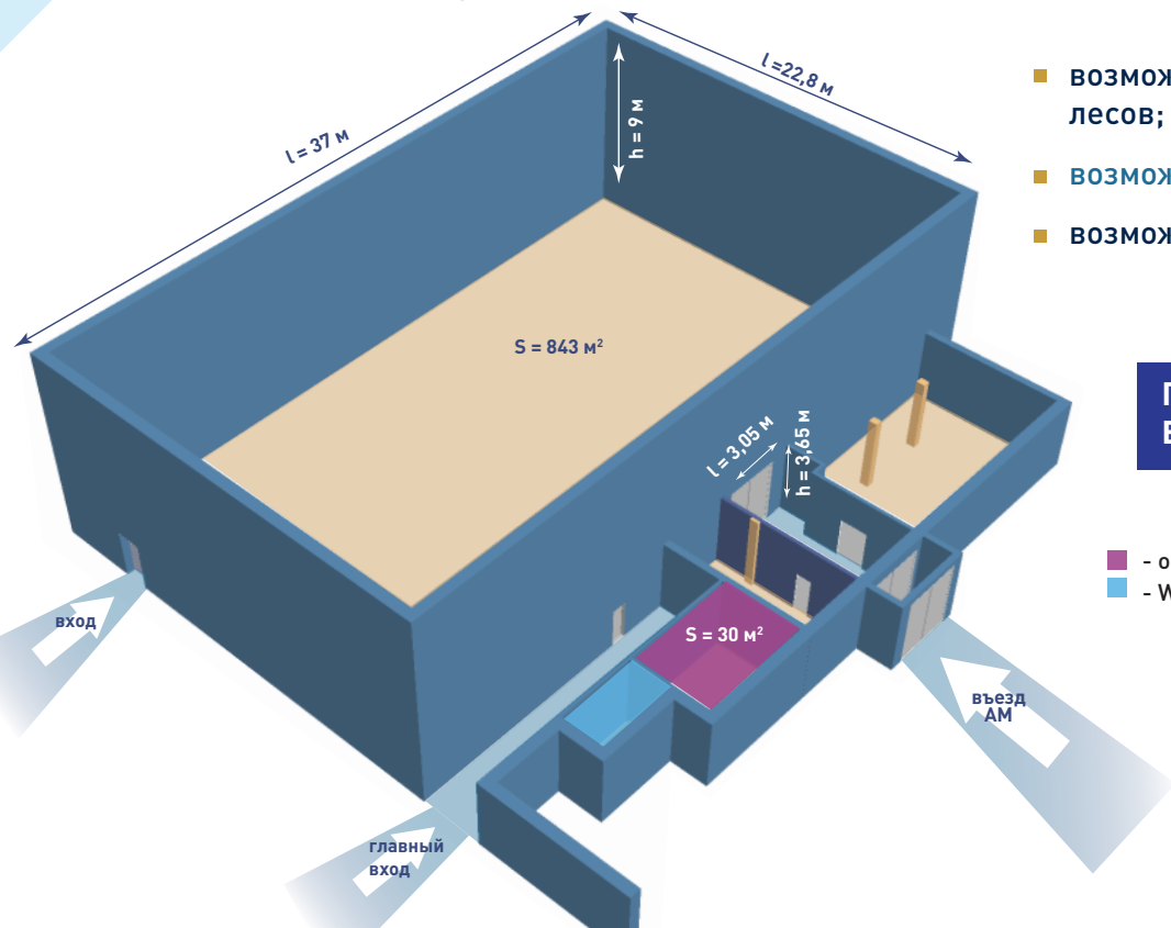
ПЛАН ПАВИЛЬОНА
