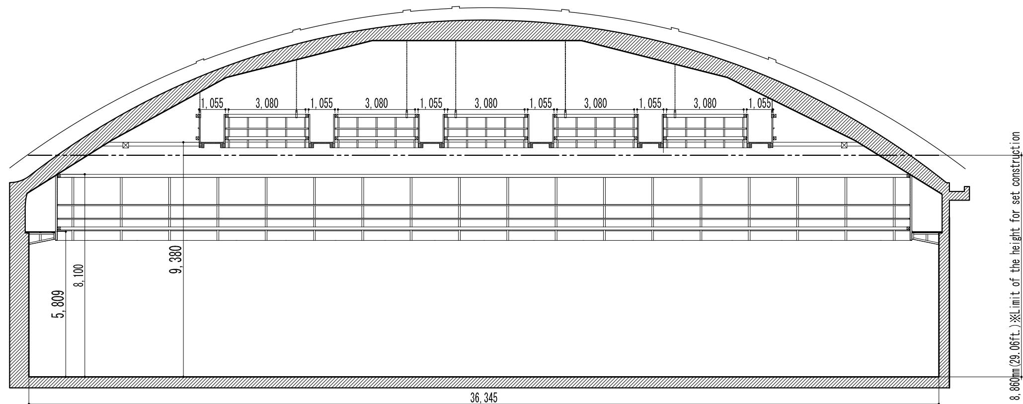
Y-Y' 断面図
