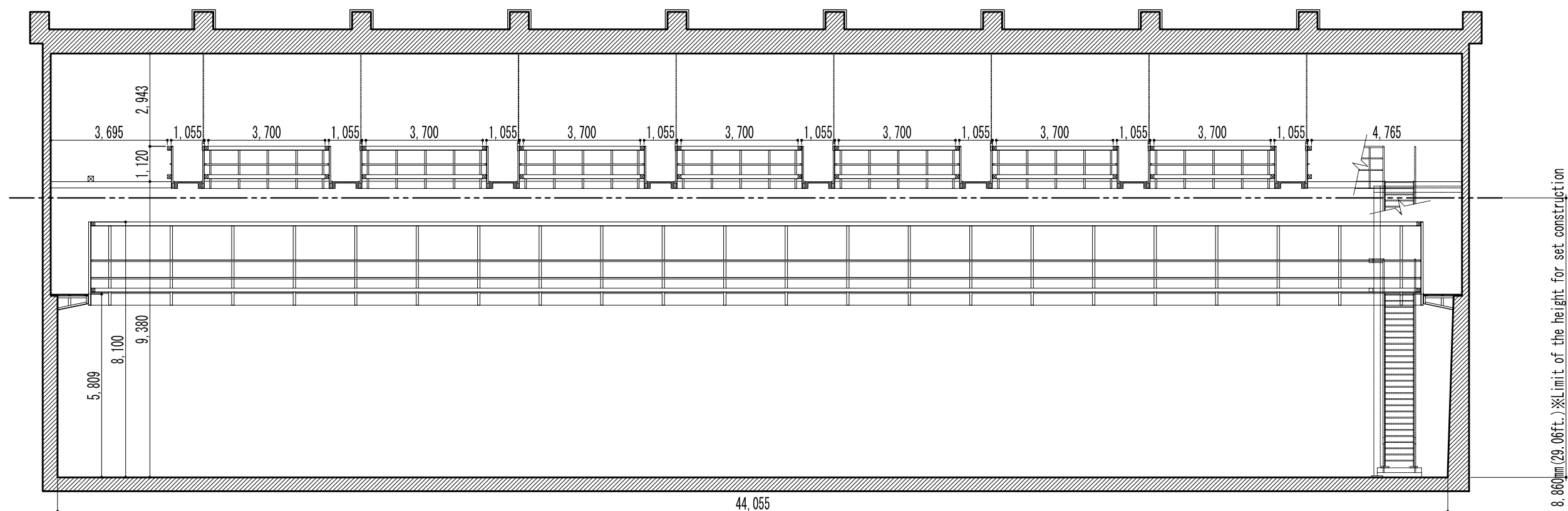
X-X' 断面図
