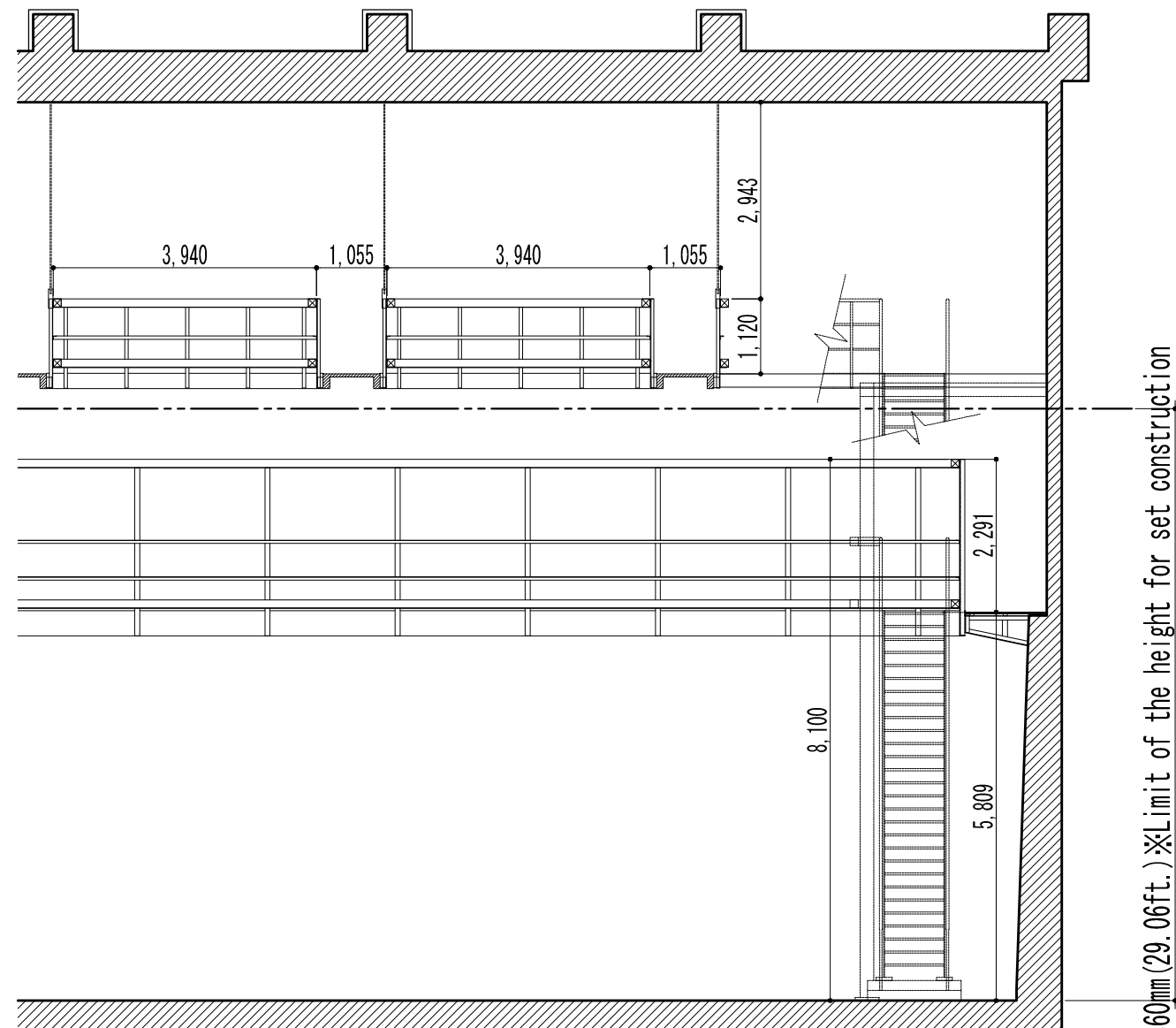
X-X' 断面図
