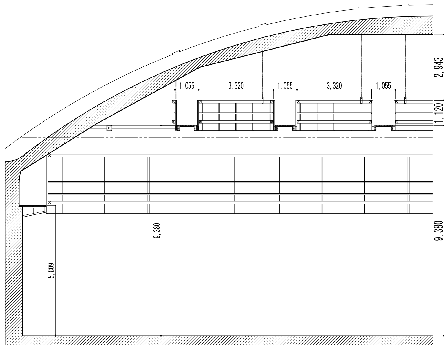
Y-Y' 断面図
