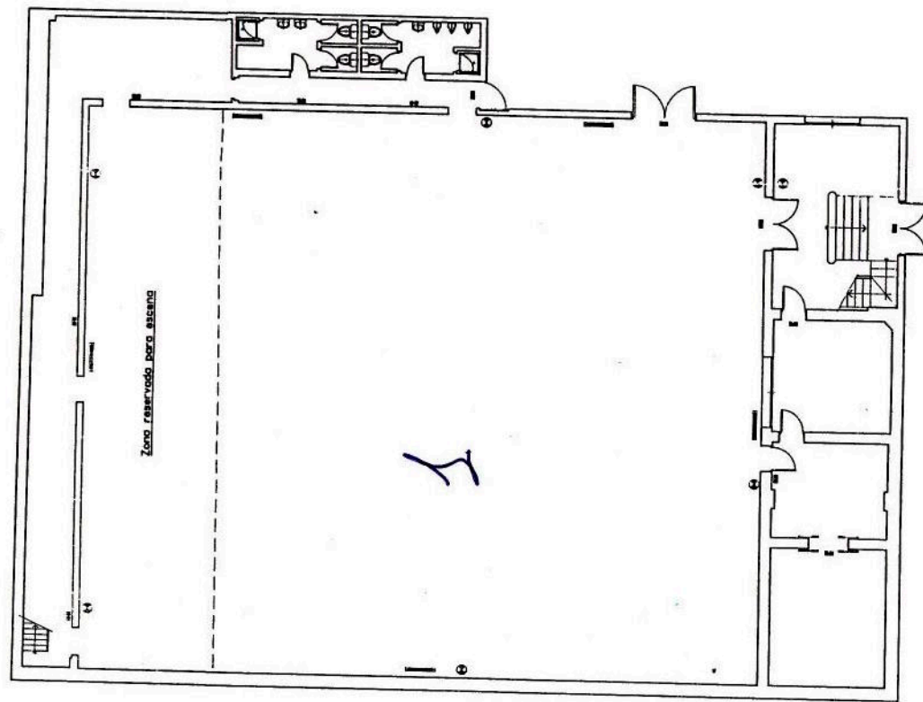
PLANTA BAJA
