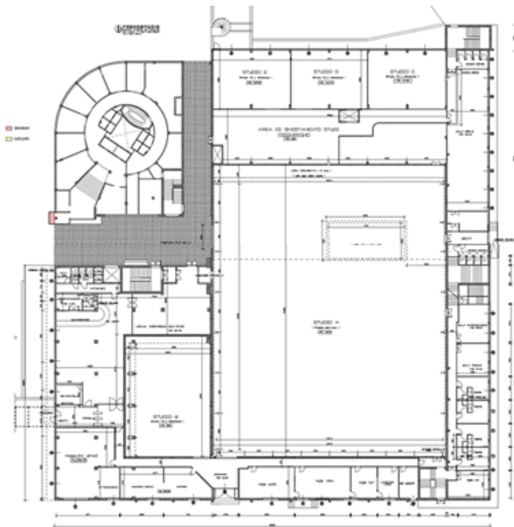
PIANTA PIANO TERRA DI PROGETTO - QUOTA 0.00
